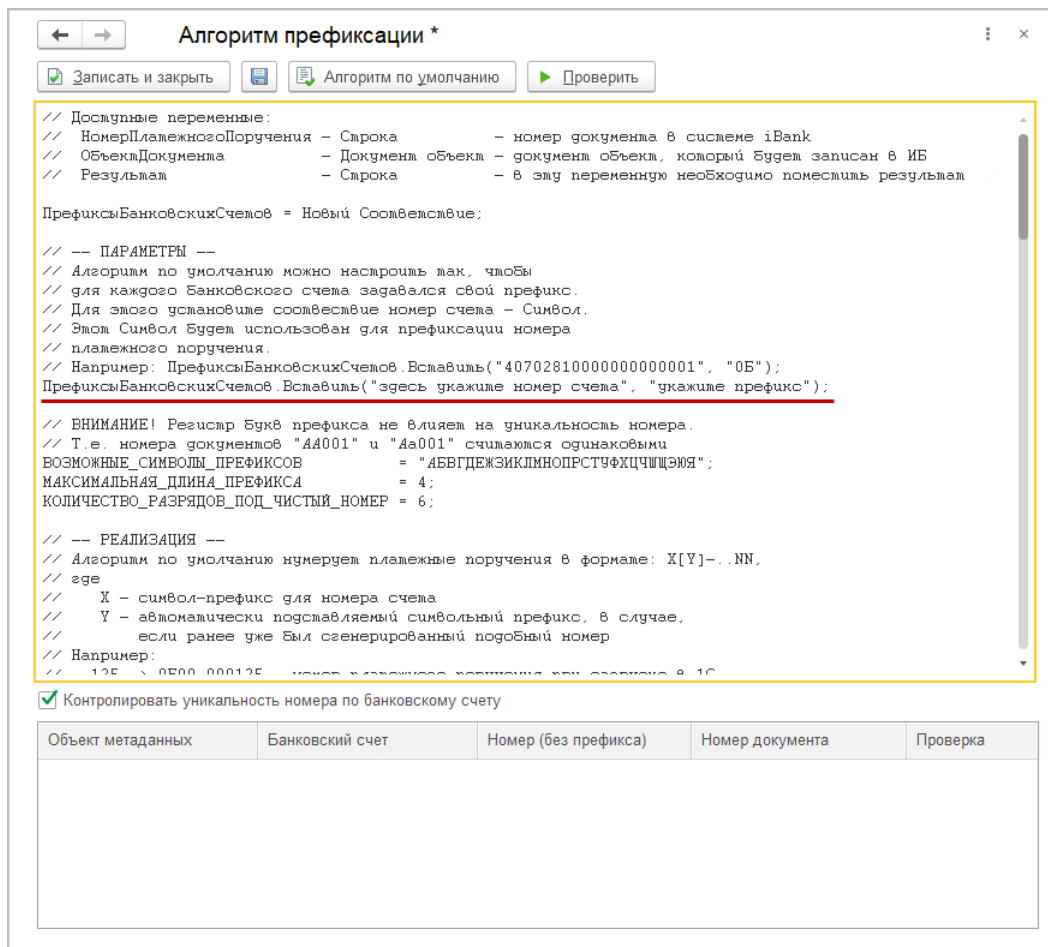
Рис. 31. Форма для ввода пользовательского алгоритма префиксации
